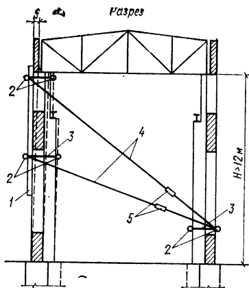
Рис. 15. Крепление отклонившейся или выпучившейся стены стальными стяжками (расчалками)
