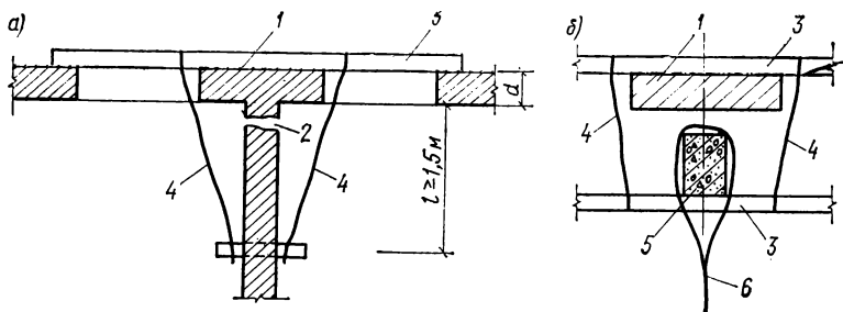
Рис. 18. Крепление отклонившихся или выпучившихся стен хомутами-скрутками a — к поперечной стене; б — к колонне; 1 — простенок; 2 — трещина; 3 — поперечина диаметром 16—18 см; 4 — проволочная скрутка диаметром 5—6 мм; 5 — колонна; 6 — растяжка или расчалка диаметром 16 мм
