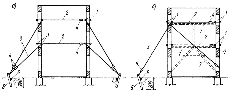
Рис. 16. Крепление стен растяжками
