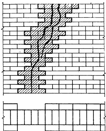
Рис. 9. Заделка трещин с разборкой старой кладки
