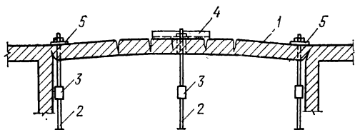
Рис. 7. Крепление выпуклой стены металлическими тяжами
