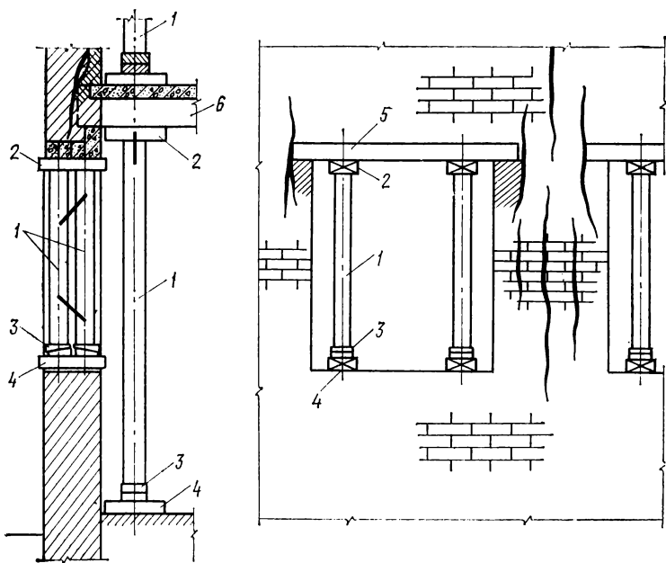
Рис. 5. Укрепление и разгрузка от массы перекрытий поврежденных простенков стойками 1 — стойка; 2 — подкладка; 3 — клинья; 4 — лежень; 5 — перемычка; 6 — балка
