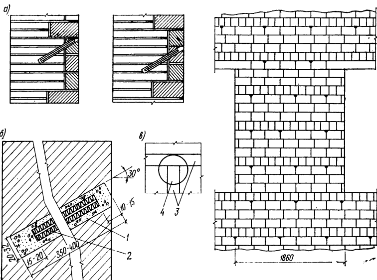
Рис. 12. Крепление поврежденной облицовки к стене
