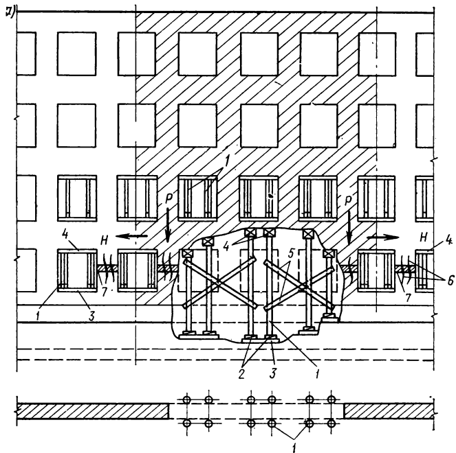
Рис. 19. Временные крепления стен
