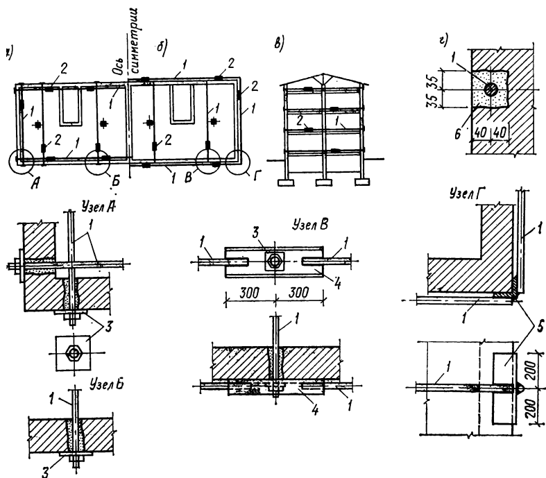
Рис. 6. Крепление стен металлическими тяжами в уровне перекрытий
