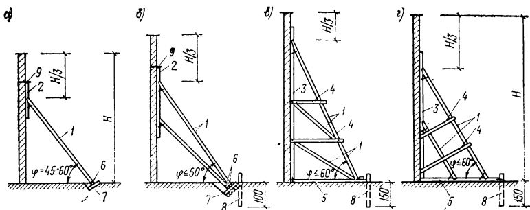
Рис. 14. Схемы крепления отклонившихся и выпучившихся стен подкосами а, б — при высоте стен до 6 м; в, г — при высоте стен 6—12 м; 1 — подкосы диаметром 16—20 см; 2 — подкладка диаметром 16—20 см; 3 — стойка диаметром 16—20 см; 4 — схватки; 5 — лежень диаметром 18—22 см; 6 — клинья; 7 — подкладка; 8 — упорный столб диаметром 18—22 см; 9 — штырь
