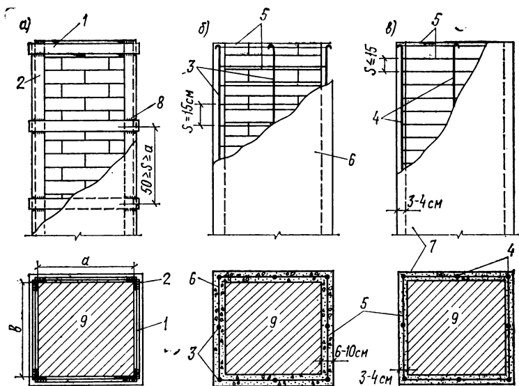
Рис. 1. Схема усиления поврежденных простенков и столбов обоймами а — стальной; б — железобетонной; в — армированной растворной; 1 — f(x) планки 35 \times 5 - 60 \times 12 мм; 2 — уголки; 3 — стержни диаметром 5—12 мм; 4 — стержни диаметром 6—12 мм; 5 — хомуты диаметром 4—10 мм; 6 — бетон марки М 150—200; 7 — раствор марки 75—100; 8 — сварка; 9 — кладка
